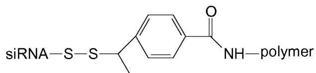
SMTP Linkage XI
