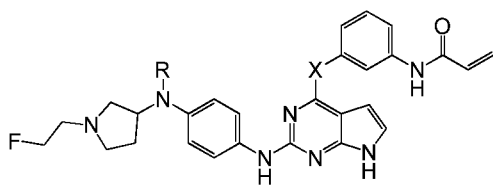
I-30 (X=O, NH, CH 2 , CF 2 ; R=H, CH 3 )
