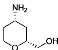
cis-(4-aminotetrahydro-2 H -pyran-2-yl)methanol
