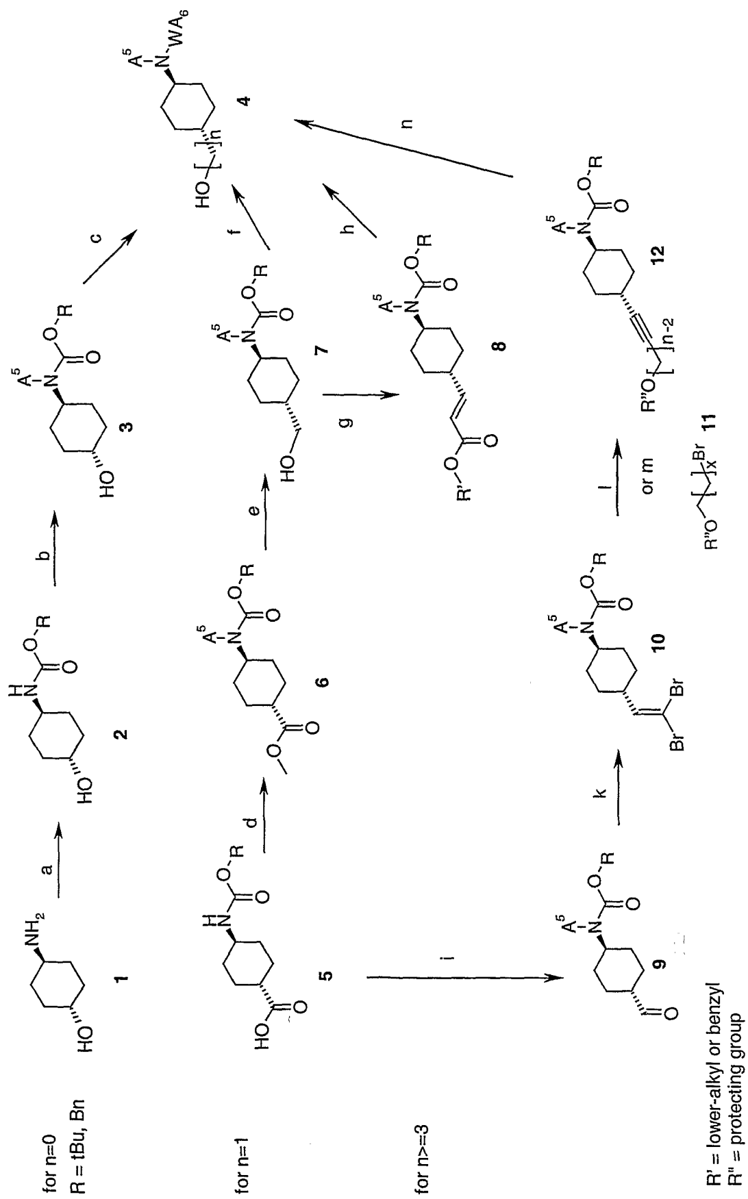
Scheme 1a
