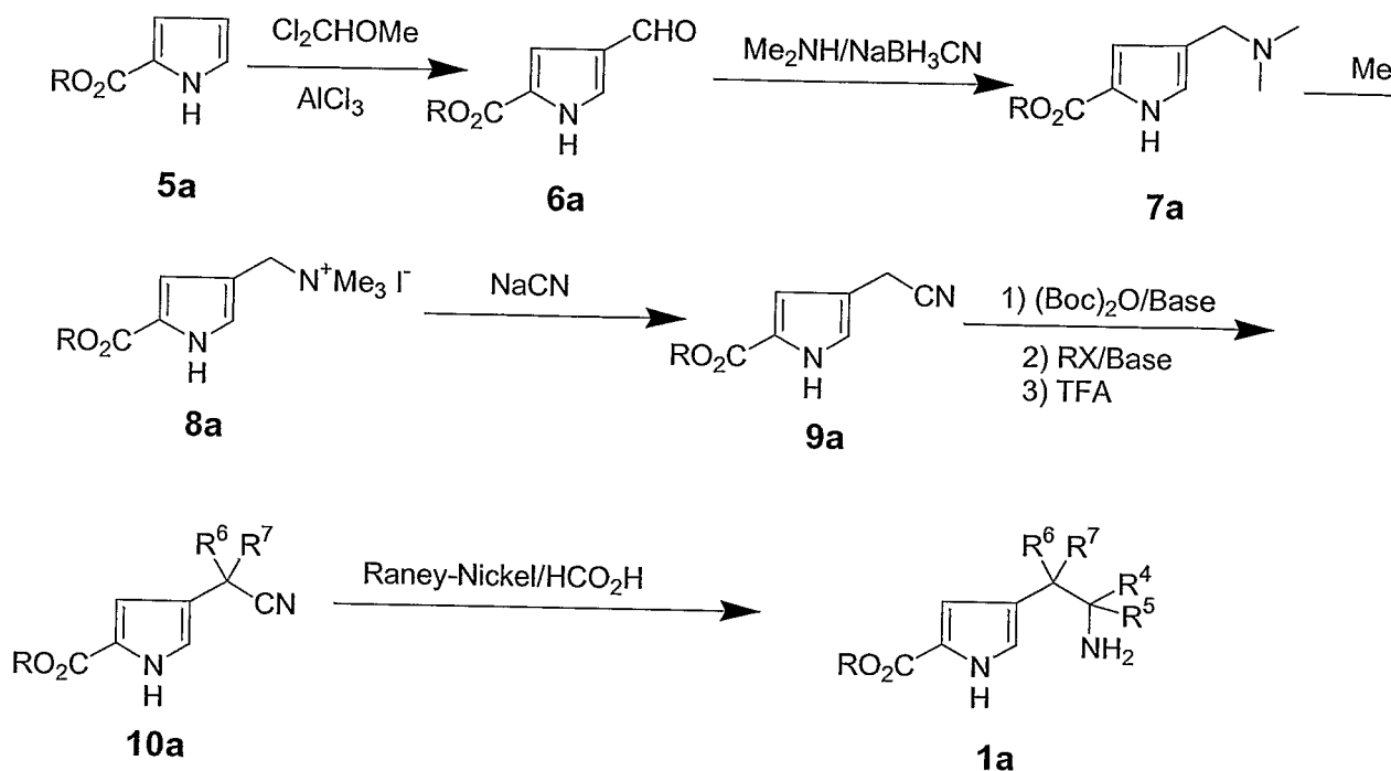
SCHEME 2A
