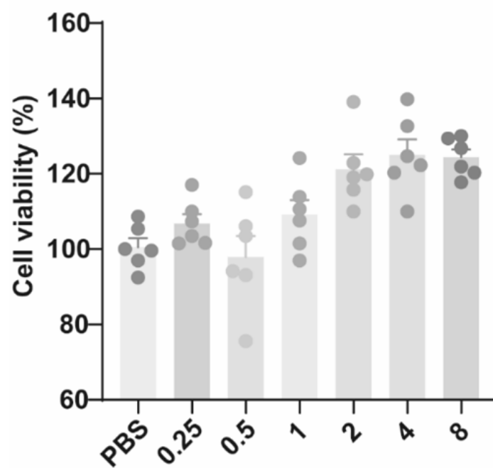
Fig. 13 CCK-8
