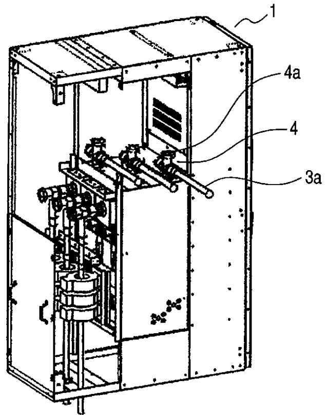
FIG. 6A
