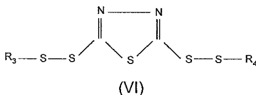
2,5-bis(hydrocarbyldithio)-1,3,4-thiadiazole
