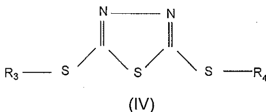
2,5-bis(hydrocarbylthio)-1,3,4-thiadiazole
