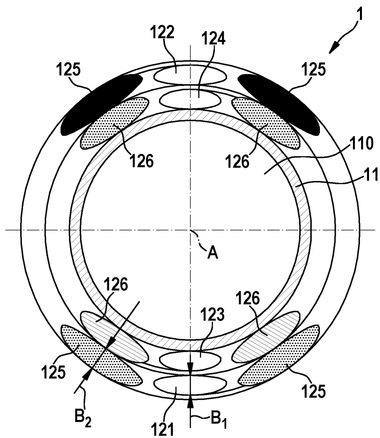
FIG. 4 (A-A)
