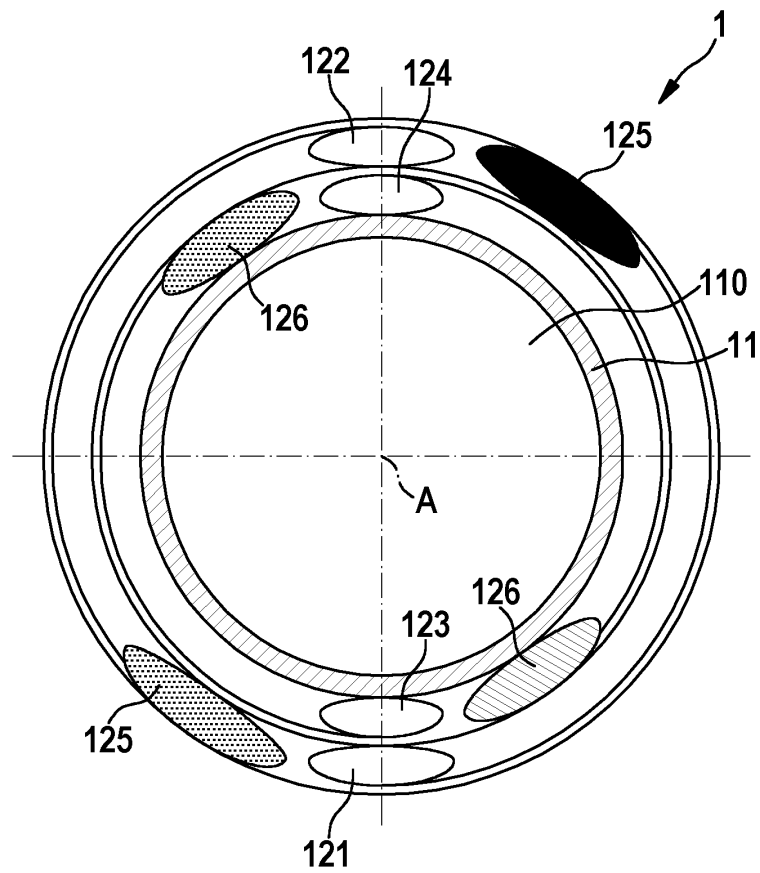
FIG. 6 (B-B)
