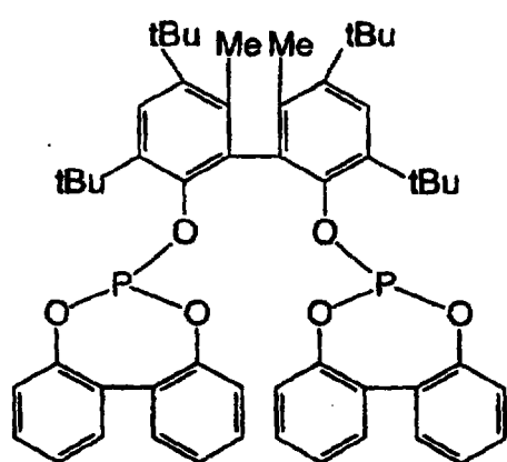
Ligand Y
