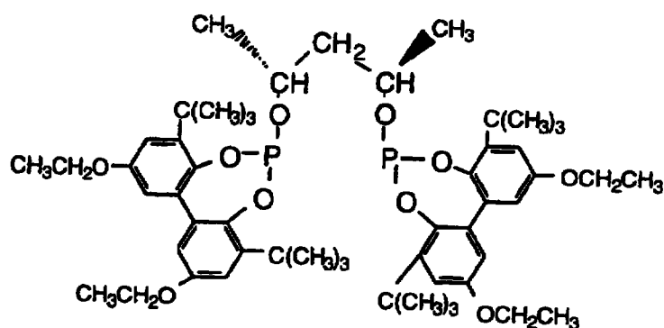
Ligand K
