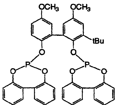
Ligand W
