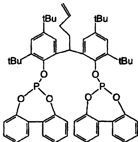
Ligand Z
