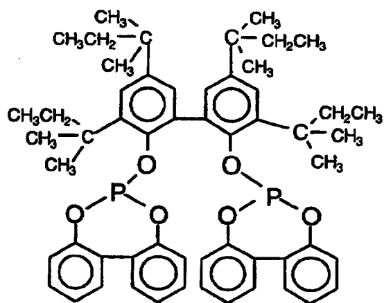
Ligand E
