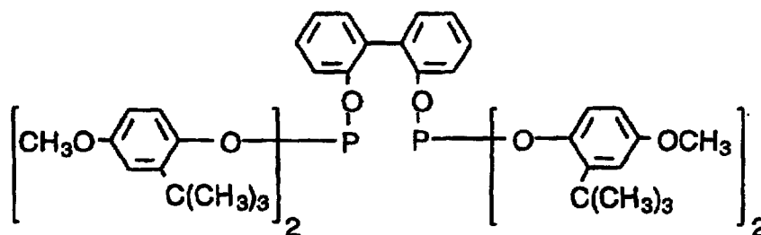
Ligand V
