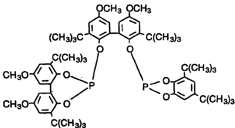
Ligand N
