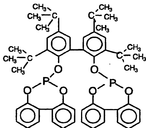
Ligand F
