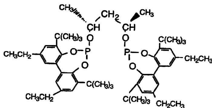
Ligand L
