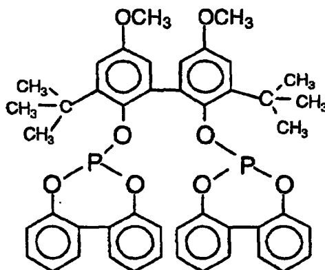
Ligand D
