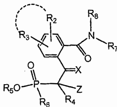
Formula (D)
