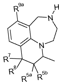
I.zz
