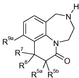
I.j
