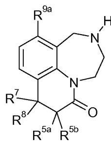
I.l
