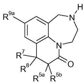
I.k
