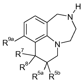
I.g
