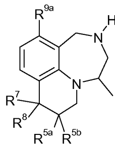
I.u
