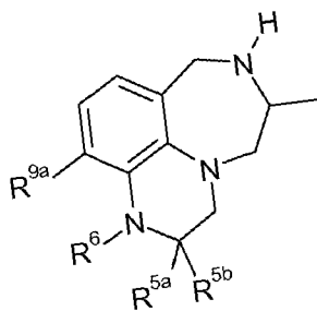
I.dd
