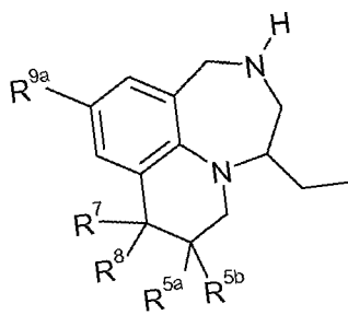
I.w
