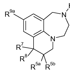
I.h
