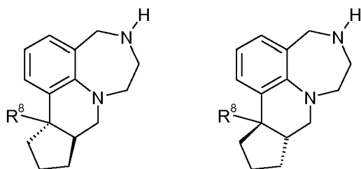
(I.1.3-trans)
