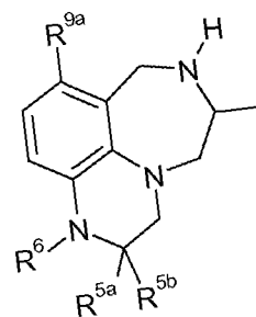
I.ff
