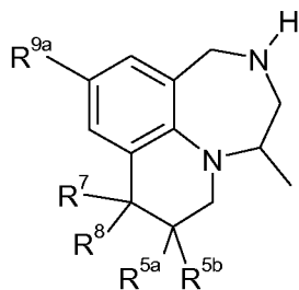
I.t
