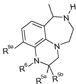
I.aa
