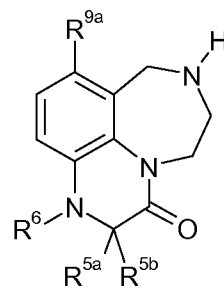
I.f
