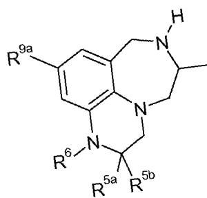
I.ee
