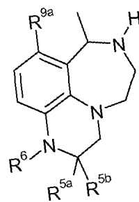
I.cc
