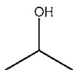
2-propanol
