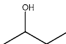
2-butanol
