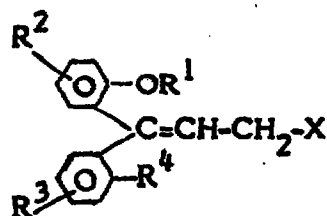
VIIa
