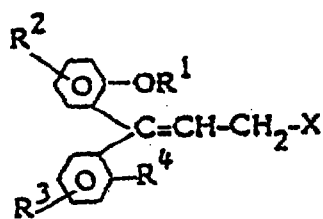
VIIa
