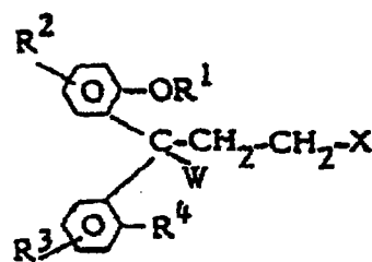
VIIb
