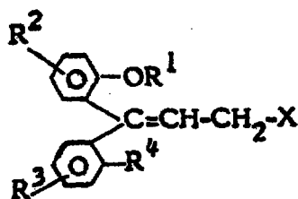
VIIa
