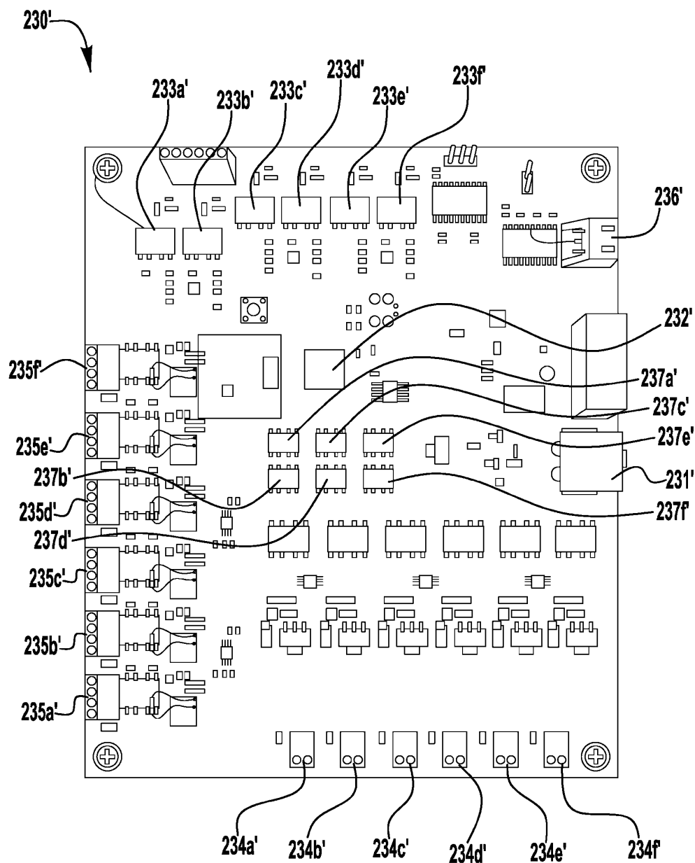
FIG. 3A
