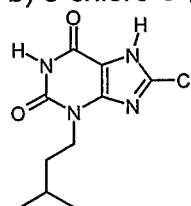
b) 8-chloro-3-(3-methylbutyl)-3,7-dihydro-1H-purine-2,6-dione
