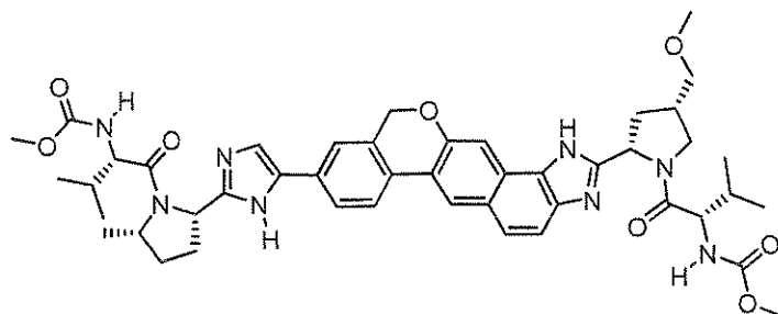
methyl ((2S)-1-((2S,5S)-2-(5-(2-((2S,4S)-1-((2S)-2-((methoxycarbonyl)amino)-3-methylbutanoyl)-4-methoxymethylpyrrolidin-2-yl)-1,11-dihydroisochromeno[4',3':6,7]naphtho[1,2-d]imidazol-9-yl)-1H-imidazol-2-yl)-5-methylpyrrolidin-1-yl)-3-methyl-1-oxobutan-2-yl)carbamate
