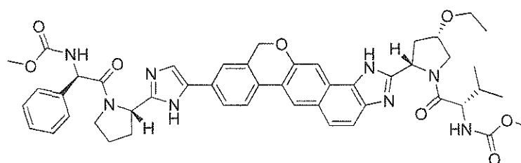
methyl ((1R)-2-[(2S)-2-(5-(2-((2S,4S)-4-ethoxy-1-((2S)-2-[(methoxycarbonyl)amino]-3-methylbutanoyl)pyrrolidin-2-yl)-1,11-dihydroisochromeno[4',3':6,7]naphtho[1,2-d]imidazol-9-yl)-1H-imidazol-2-yl)pyrrolidin-1-yl]-2-oxo-1-phenylethyl)carbamate
