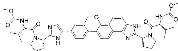
methyl ((2S)-1-[(2R)-2-(5-{2-[(2S)-1-[(2S)-2-[(methoxycarbonyl)amino]-3-methylbutanoyl]pyrrolidin-2-yl]-3,7-dihydroisochromeno[3',4':5,6]naphtho[1,2-d]imidazol-9-yl]-1H-imidazol-2-yl)pyrrolidin-1-yl]-3-methyl-1-oxobutan-2-yl]carbamate
