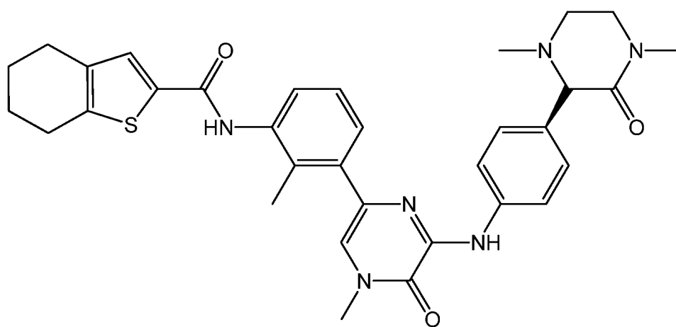
GDC-0834
