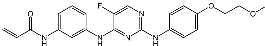
CC-292
