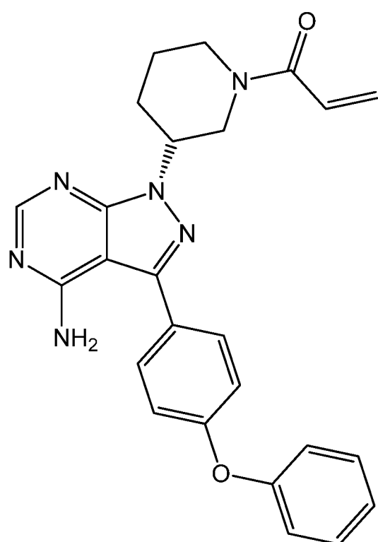
Ibrutinib
