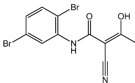
LFM-A13
