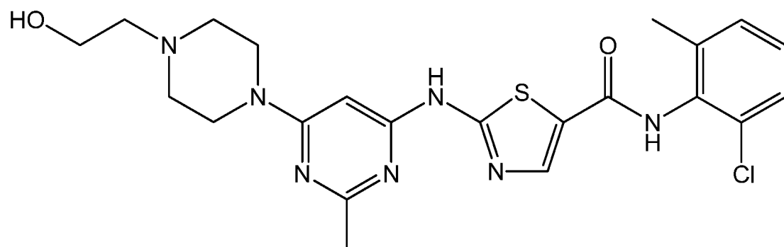
GDC-0834
