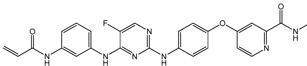
CNX-774
