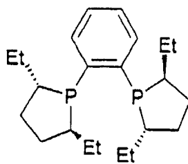
(S) -EtDuphos:
