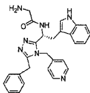
compound 171 ( R )-benzyl-3-(2-aminoisobutyramido)-3-(5-(2-(1 H -indol-3-yl)ethyl)-4-(4-methoxybenzyl)-4 H -1,2,4-triazol-3-yl)-propanoate,
