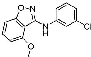
N-(3-chlorophenyl)-4-methoxybenzo[d]isoxazol-3-amine
