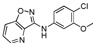
N-(4-chloro-3-methoxyphenyl)isoxazolo[4,5-b]pyridin-3-amine
