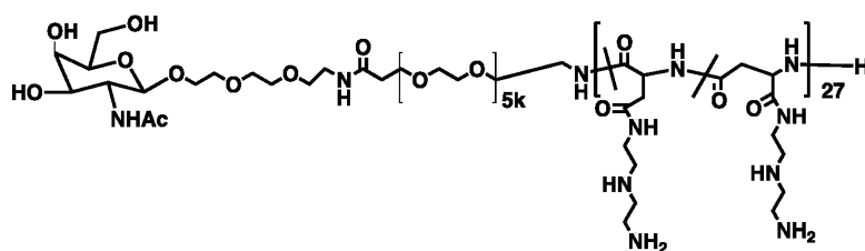
GalNAc-PEG5K-pASP(DET)
