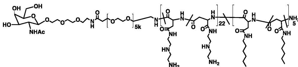
GalNAc-PEG5K-pASP(DET)-C6
