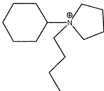
N-butyl-N-cyclohexylpyrrolidinium cation
