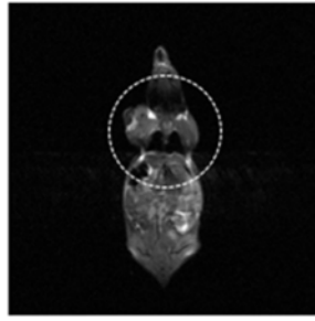
^1\text{H} MRI
