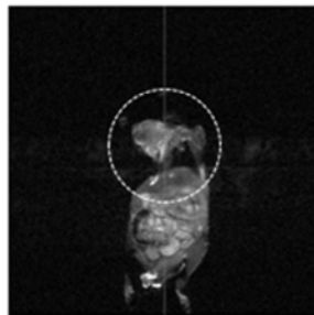
^1\text{H} MRI
