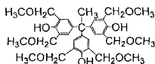
HMOM-TPHAP
