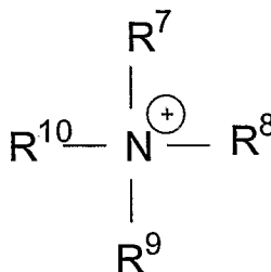
Ammonium
