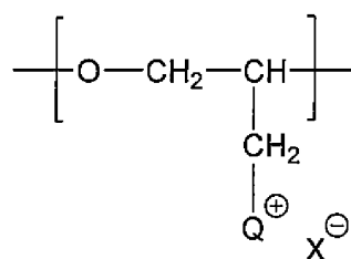
(1N)
