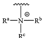
(2A)
