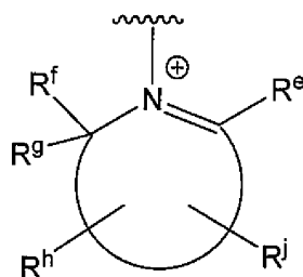
(2C)
