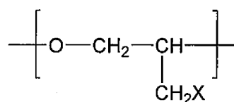
(1P)
