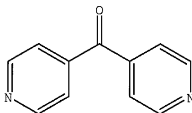
4,4'-dipyridylketone
