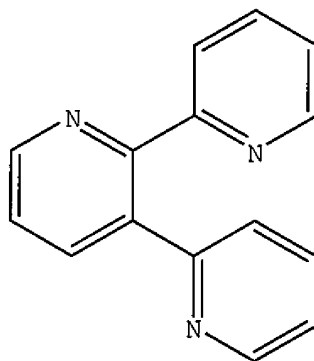
terpyridine
