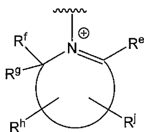
(2C)
