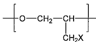
(1P)
