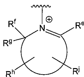
(2C)
