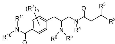
Formula (Ia);
