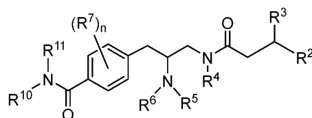
Formula (Ia);
