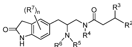
Formula (Ie);
