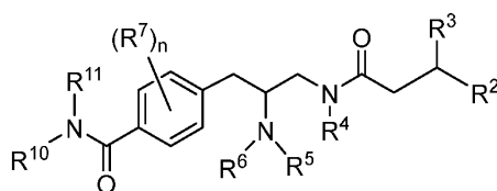
Formula (Ia);
