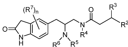
Formula (Ie);
