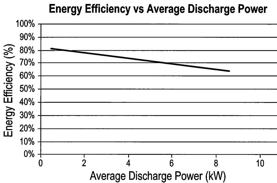
FIG. 25B
