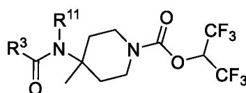
Formula (IIa);
