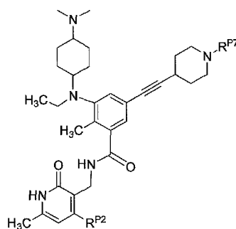
(VIIb)
