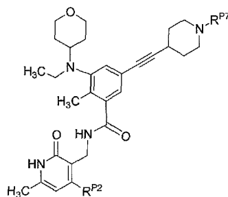
(VIIa)
