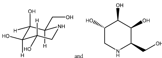
Migalastat free base
