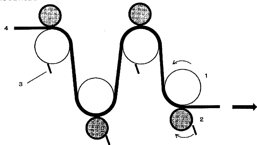
LONGITUDINAL STRETCHING DEVICE B
