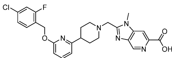
Example 2A-03
