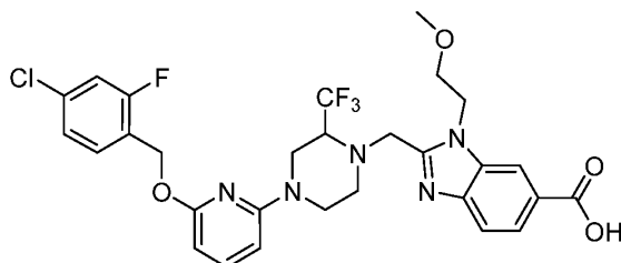
Example 12A-01
