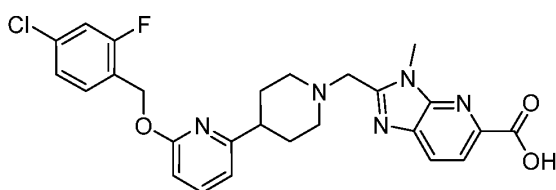
Example 2A-01
