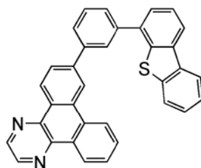
7mDBTPDBq-II
