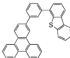
mDBTPTp-II
