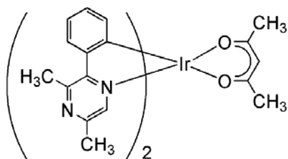
Ir(mppr-Me) 2 acac
