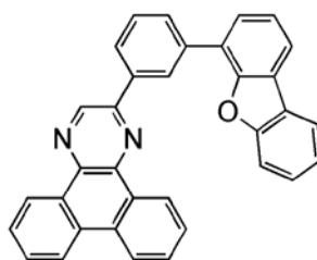
2mDBFPDBq-II
