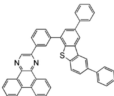
2mDBTPDBq-III
