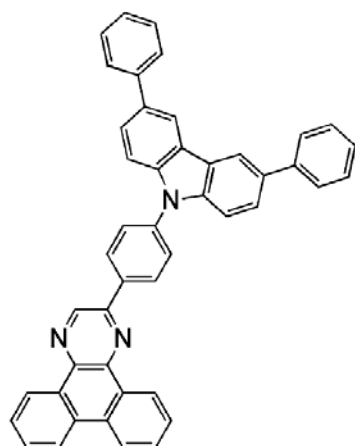
2CzPDBq-III
