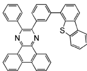
3Ph-2mDBTPDBq-II
