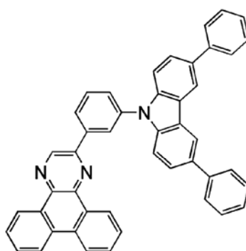
2mCzPDBq-III
