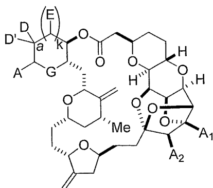
halichondrin macrolide
