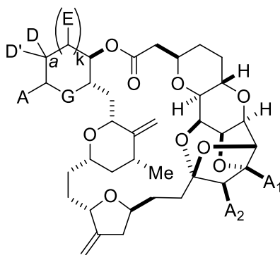
halichondrin macrolide
