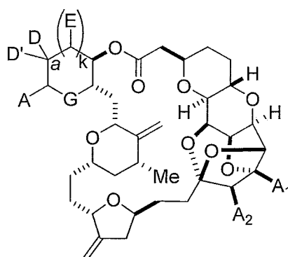
halichondrin macrolide
