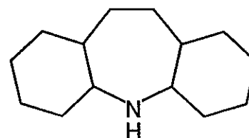
Perhydroiminostilbene
