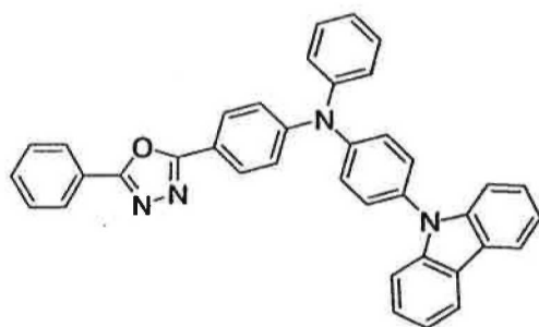
YGAO11
