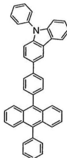
PCzPA
