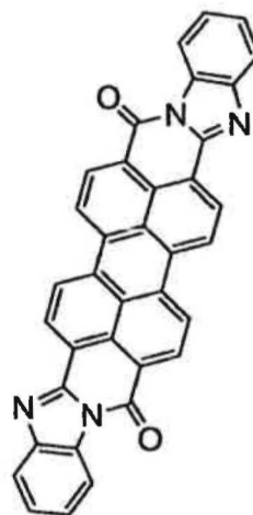
PTCBI
