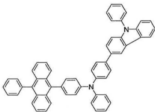
PCBAPA
