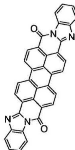
PTCBI
