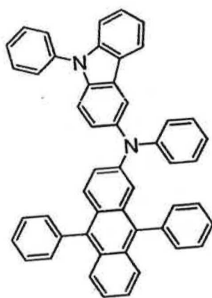
2PCAPA
