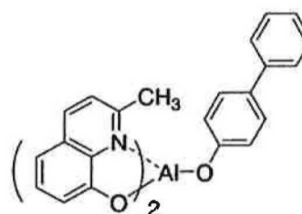
BAlq
