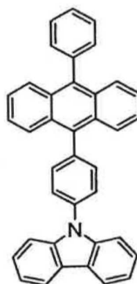
CzPA
