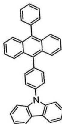
CzPA
