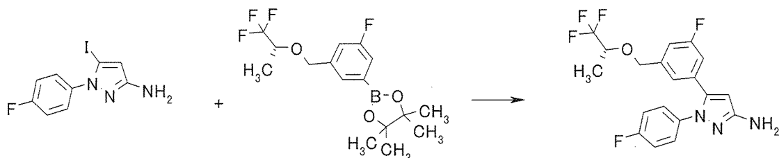
(1) 1-(4-Fluorophenyl)-5-[3-fluoro-5-((R)-2,2,2-trifluoro-1-methylethoxymethyl)phenyl]-1H-pyrazol-3-ylamine
