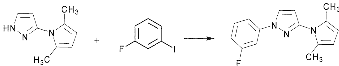
(2) 3-(2,5-Dimethylpyrrol-1-yl)-1-(3-fluorophenyl)-1H-pyrazole
