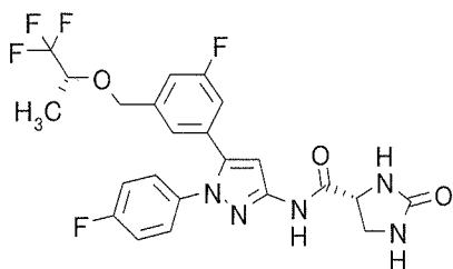
(1) 1-(4-Fluorophenyl)-5-[3-fluoro-5-((R)-2,2,2-trifluoro-1-methylethoxymethyl)phenyl]-1H-pyrazol-3-ylamine
