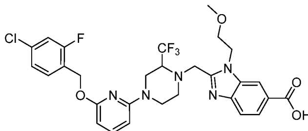
Example 12A-01
