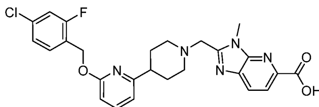
Example 2A-01
