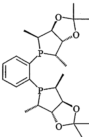
( S,S,S,S )-"Me-KetalPhos",
