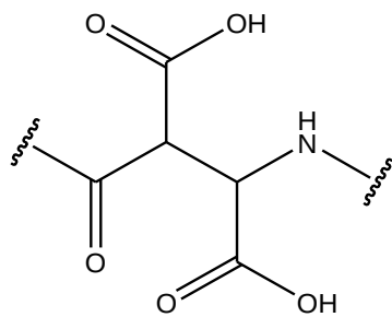
(β Lym)
