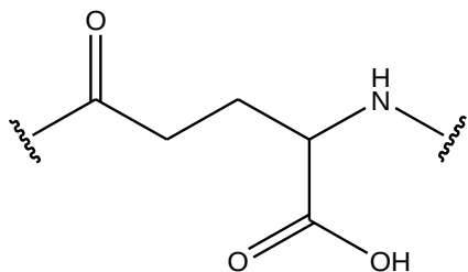
(γ Glu)
