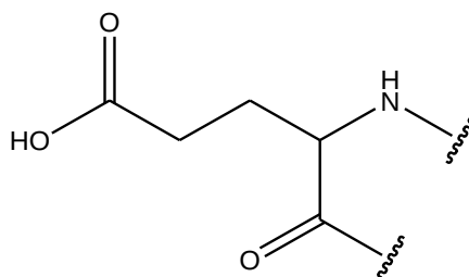
(Glu)
