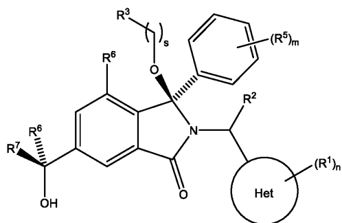
Diastereoisomer 2A
