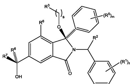
Diastereoisomer 2A
