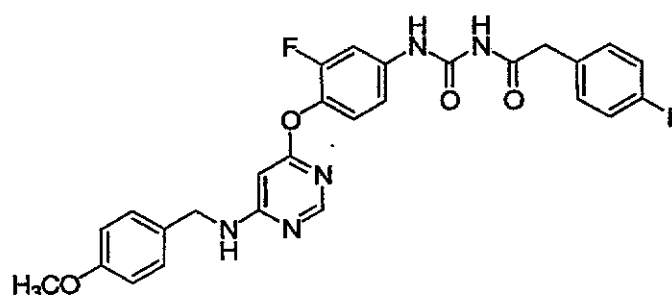
1-(4-(6-(4-Methoxybenzylamino)pyrimidin-4-yloxy)-3-fluorophenyl)-3-(2-(4-fluorophenyl)acetyl)urea
