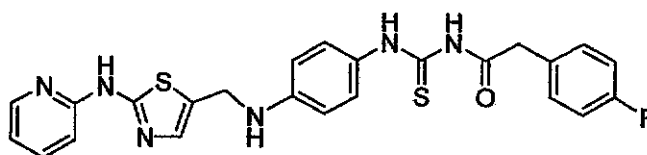
1-(2-(4-Fluorophenyl)acetyl)-3-(4-((2-(pyridin-2-ylamino)thiazol-5-yl)methylamino)phenyl)thiourea
