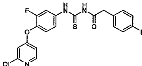
1-(4-(2-Chloropyridin-4-yloxy)-3-fluorophenyl)-3-(2-(4-fluorophenyl)acetyl)thiourea
