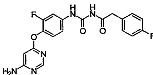
1-(4-(6-Aminopyrimidin-4-yloxy)-3-fluorophenyl)-3-(2-(4-fluorophenyl)acetyl)urea
