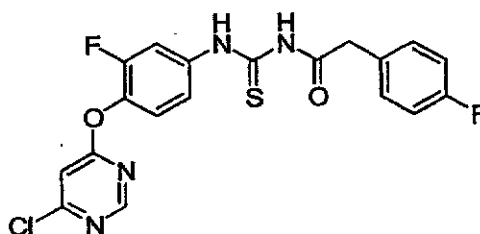
10 1-(4-(6-Chloropyrimidin-4-yloxy)-3-fluorophenyl)-3-(2-(4-fluorophenyl)acetyl)thiourea
