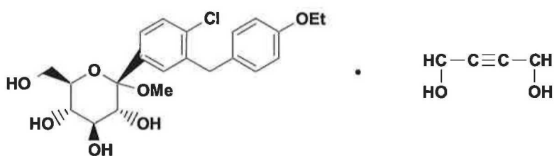
If
