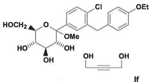
If
