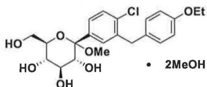
Ig
