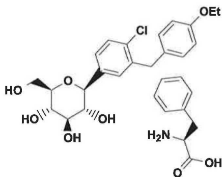
Compound Ik
