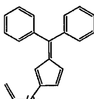
2-(but-3-enyl)-6,6-diphenylpentafulvene
