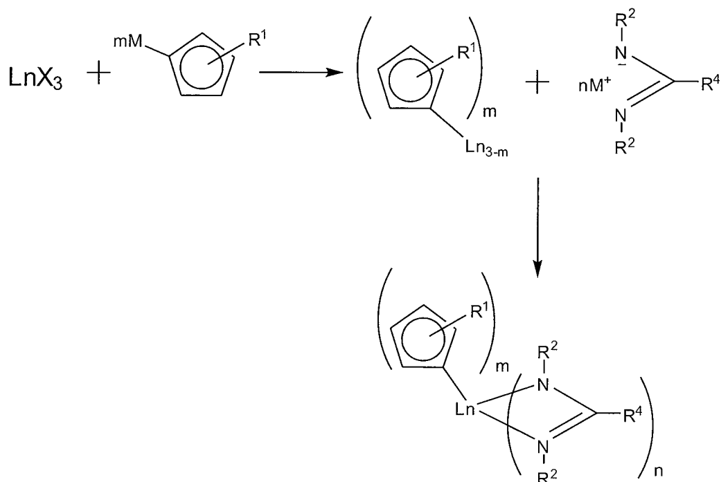
Scheme-3
