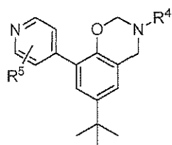
IIA-3, or
