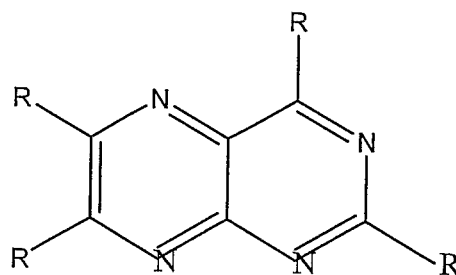
Pteridine
