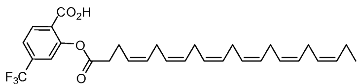
VIg-2
