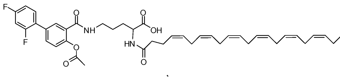
IVb-7
