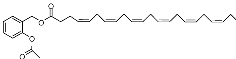
Ie-2
