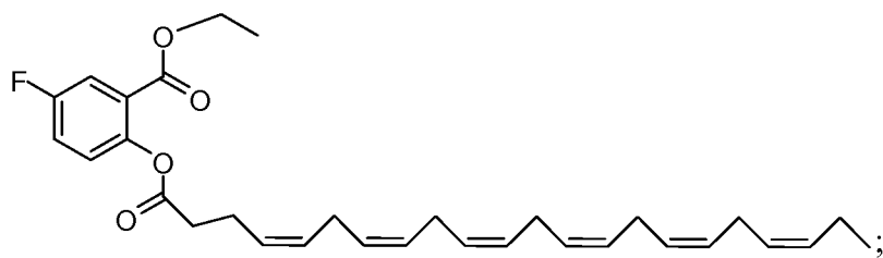
Id-5
