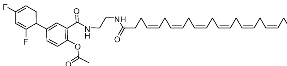
IVb-11
