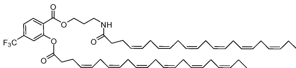
VIc-6
