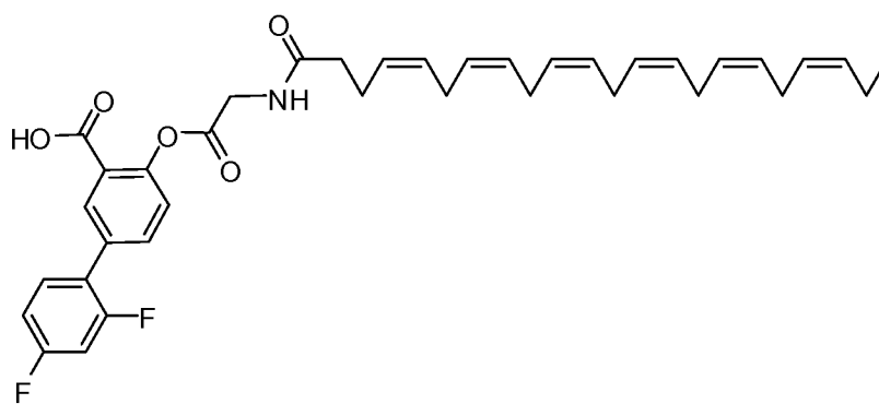
IVf-1
