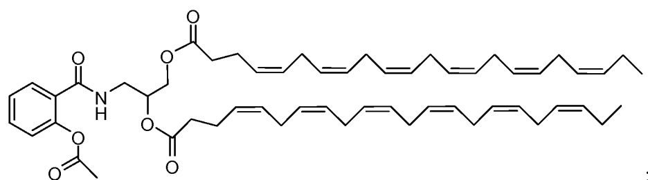
Ic-3
