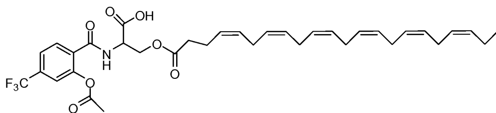
VIb-11
