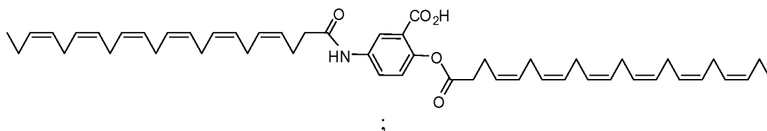
III-8
