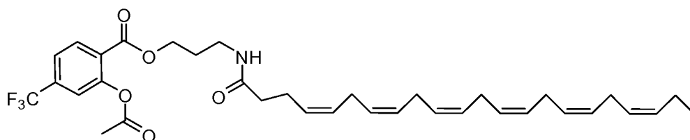
VIb-2
