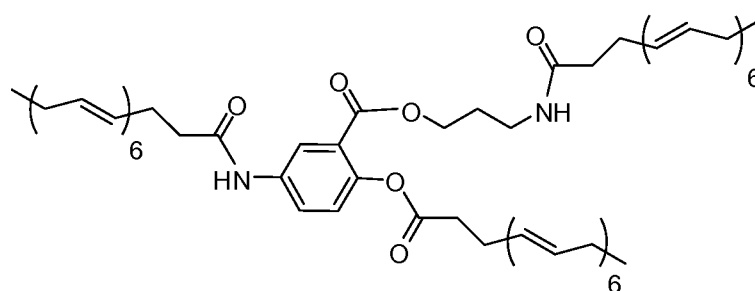
III-9
