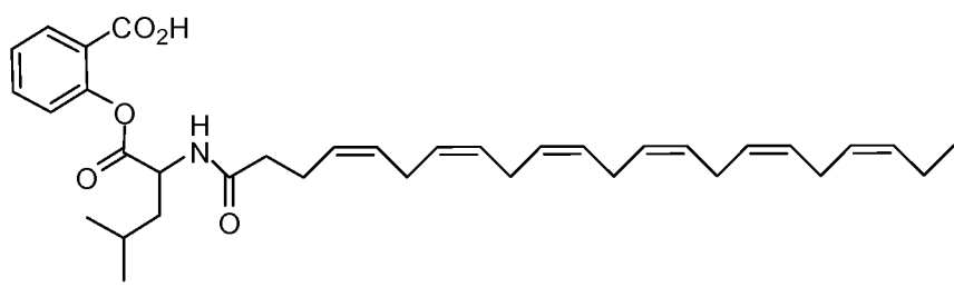
Ig-1
