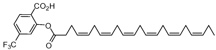
VIa-1
