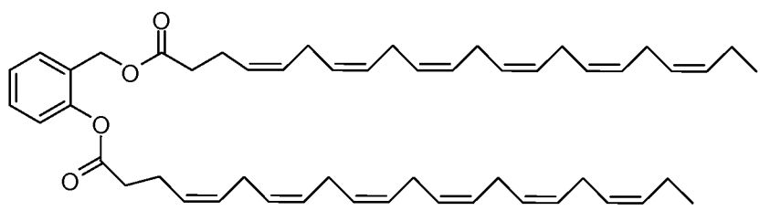
Ie-1
