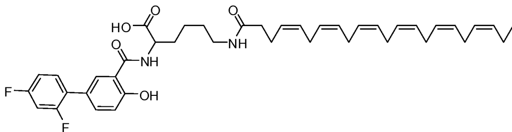
IVc-5
