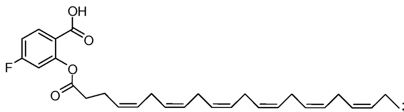
Ia-3
