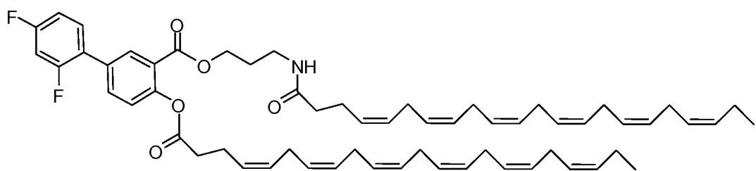
IVc-5
