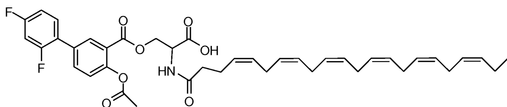
IVb-9
